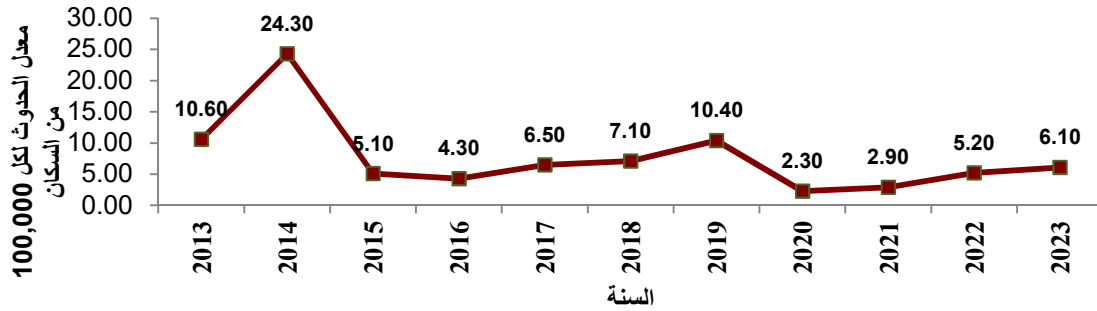
الرسم البياني (27) معدل الإصابة بالتهاب السحايا البكتيري (أخرى) لكل 100,000 من السكان، فلسطين 2023 - 2013
