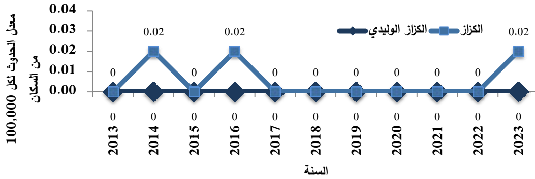
الرسم البياني (25) معدل الإصابة بالكزاز لكل 100,000 من السكان، فلسطين 2013-2023
